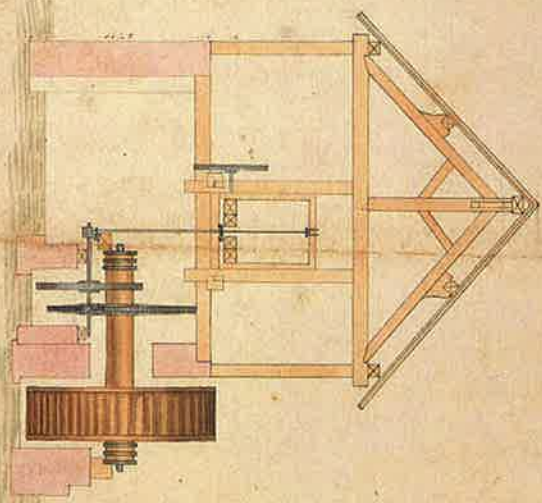
Coupe en bois
