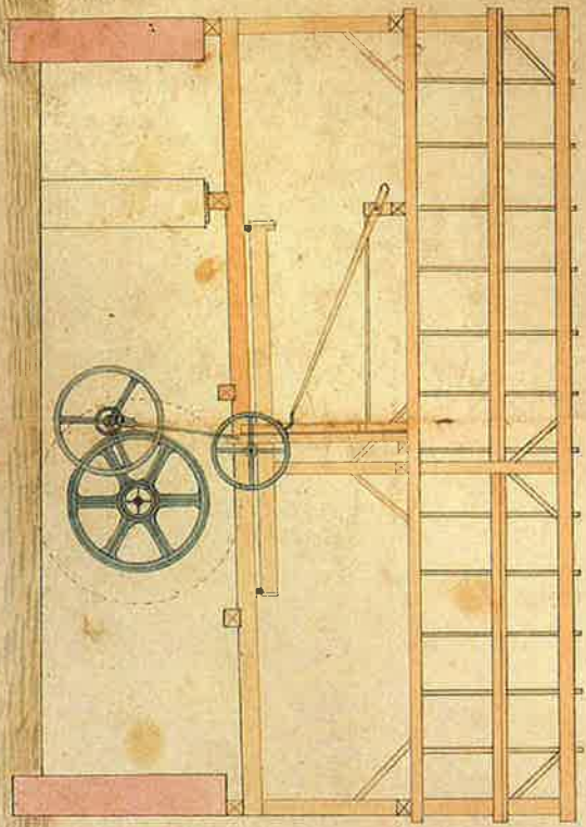
Coupe en fer
