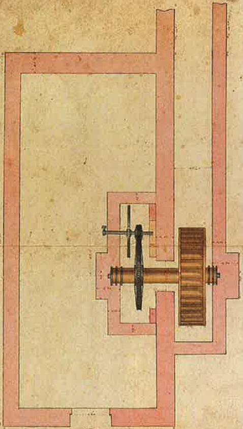
Plan en bois
